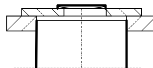
zwieńczenie - pierścień odciążający, płyta nastudzienna, właz żeliwny
