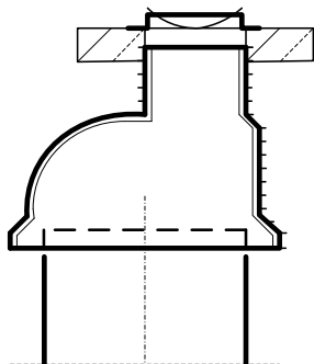
zwieńczenie - stożek, płyta nastudzienna, właz żeliwny
